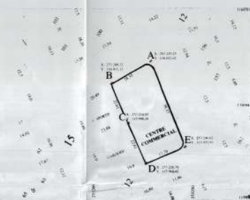
Plan de masse ech: 1/500
