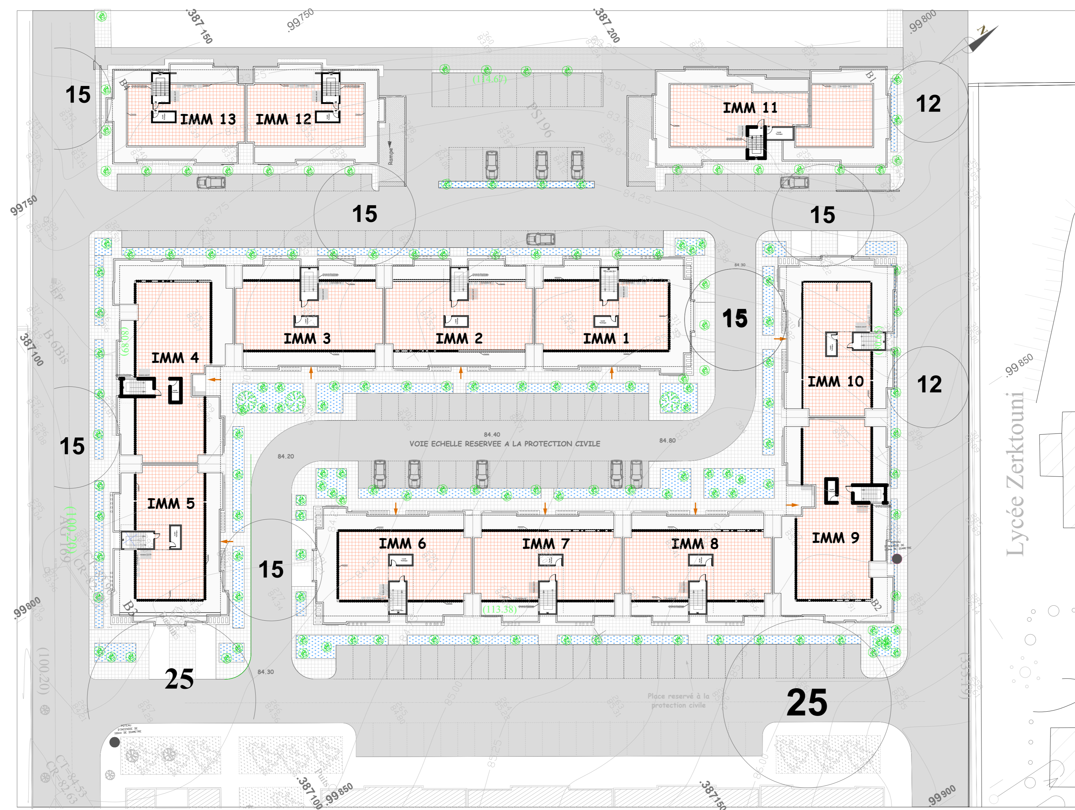
PLAN DE MASSE
