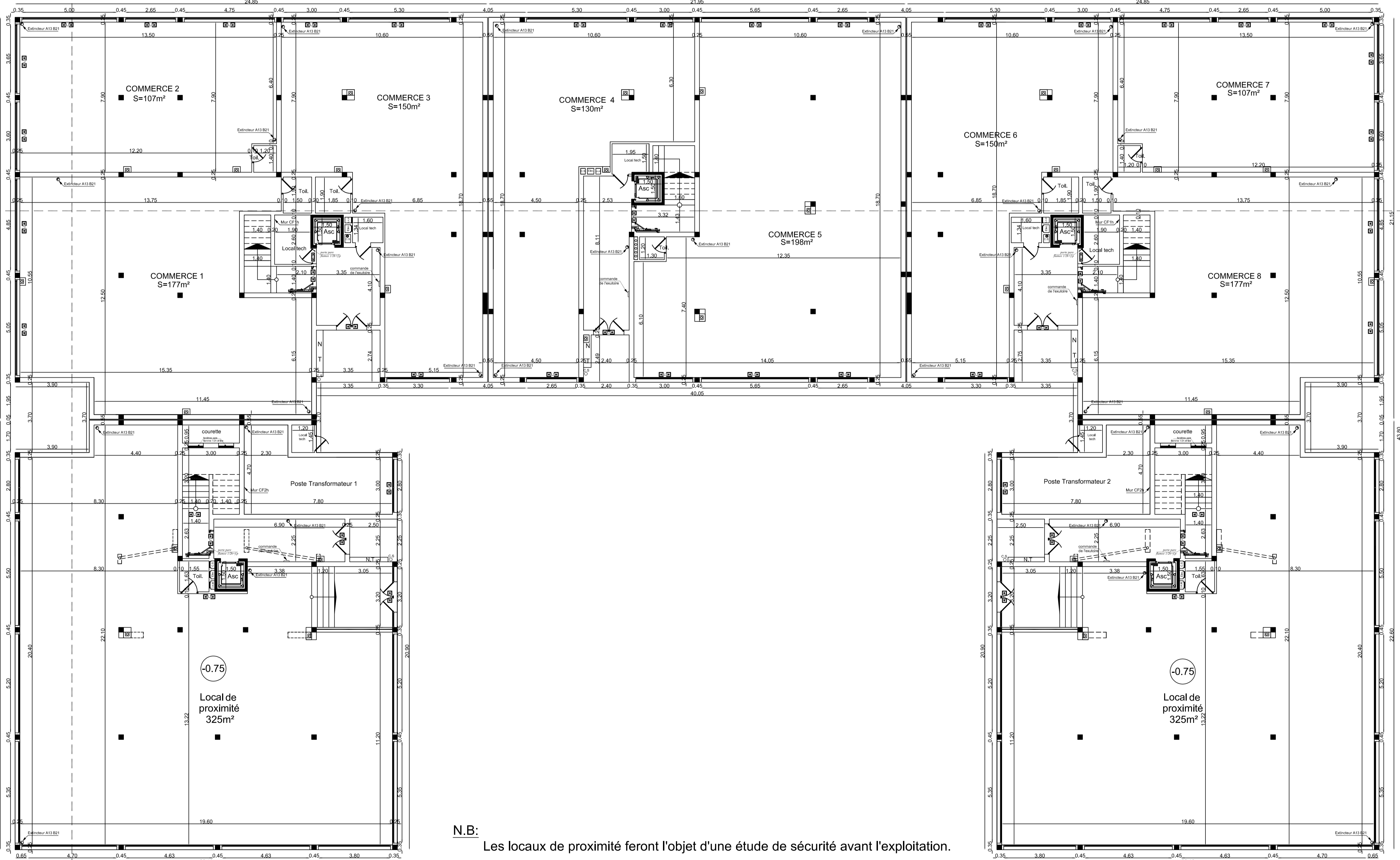
REZ DE CHAUSSEE
